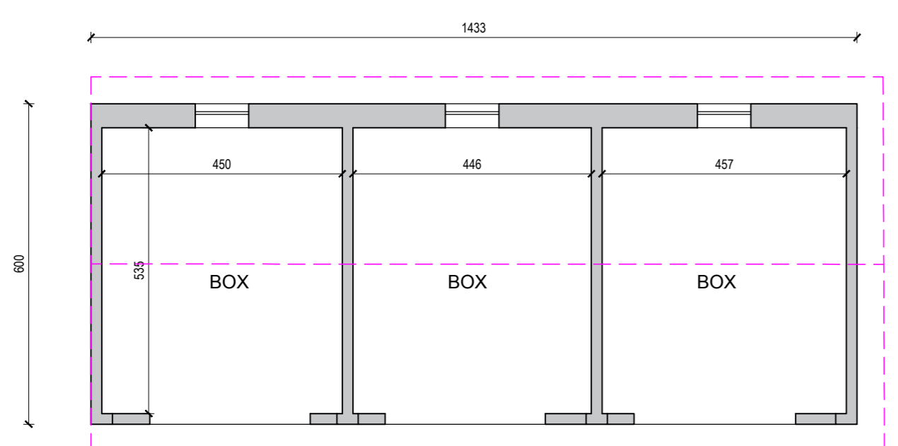
PIANTA EDIFICIO "BASSO"
