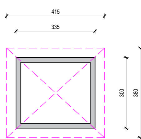
PIANTA CABINA ENEL
